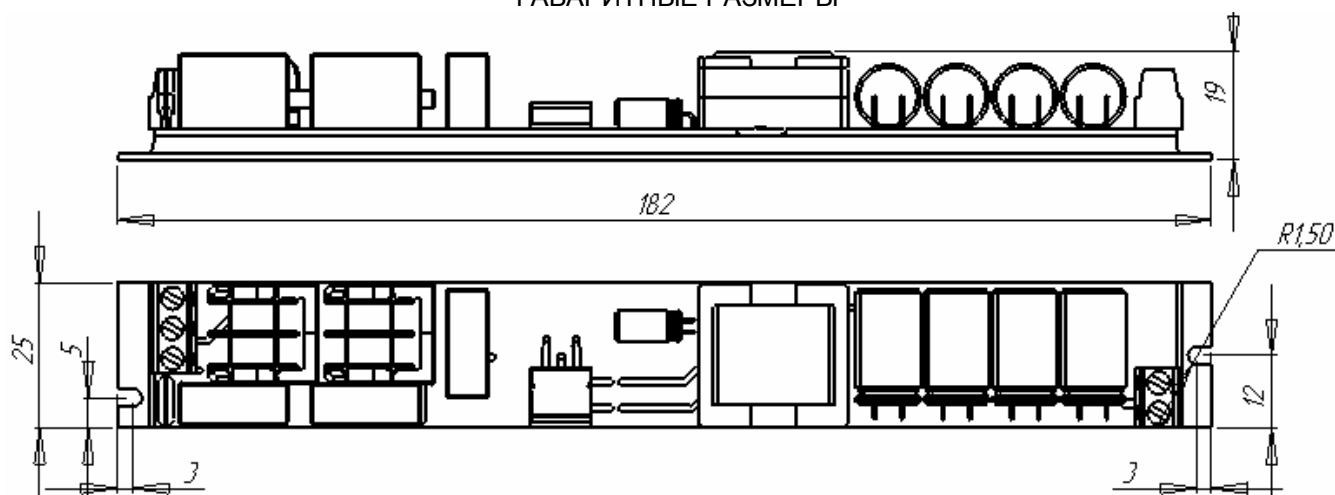
Рис. 2 Размеры блока в исполнении с заливкой
